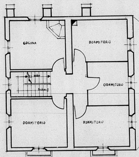
PLANTA 1ª
