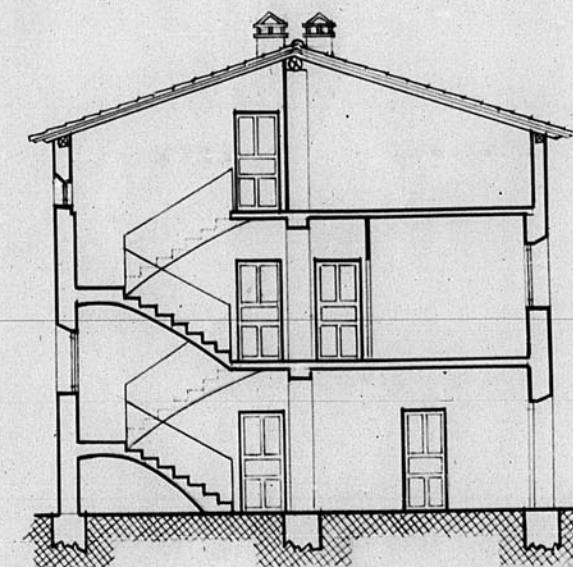
SECCION
