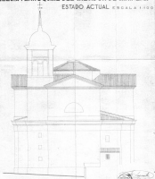
ALCEGO POSTERIOR
