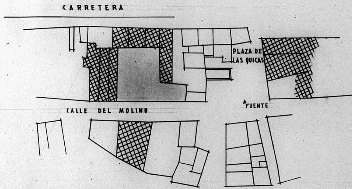
Plano de emplazamiento Escala 1:1000
