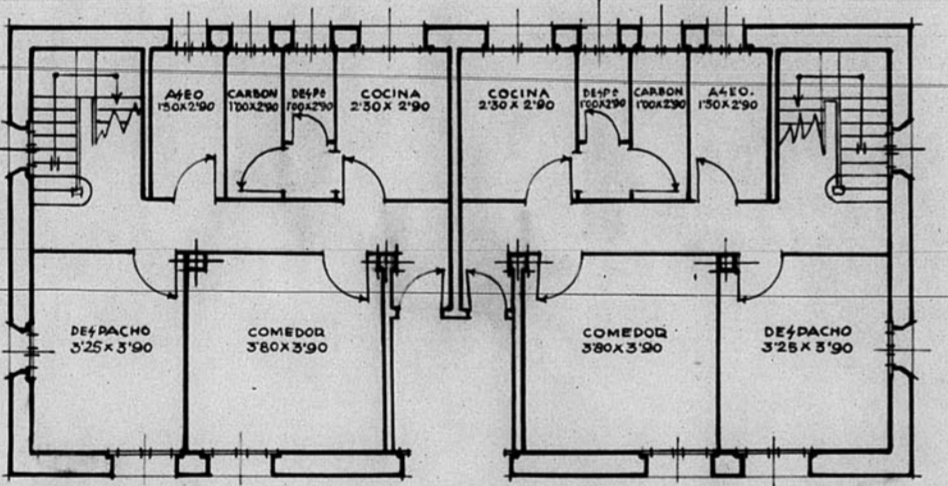
Planta baja.
