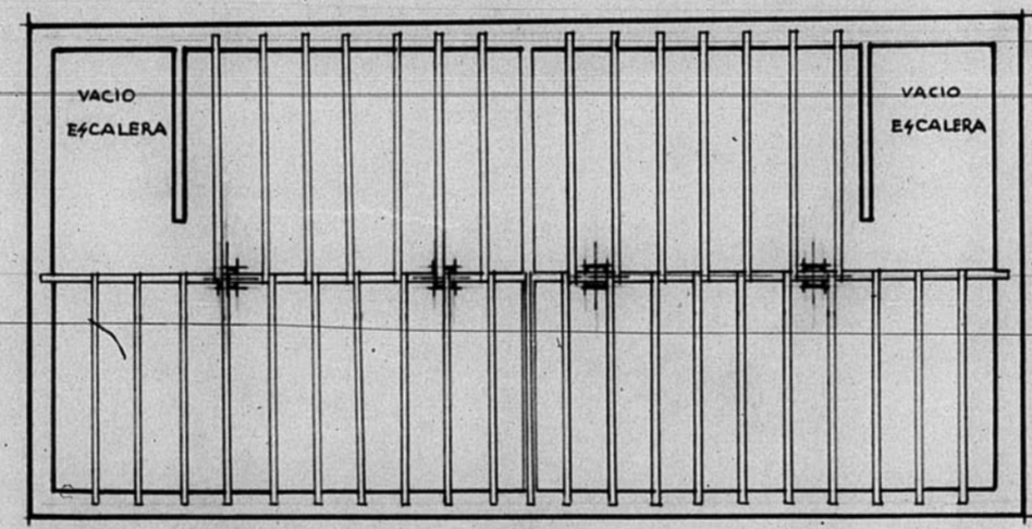
Planta de entramado de pisos.
