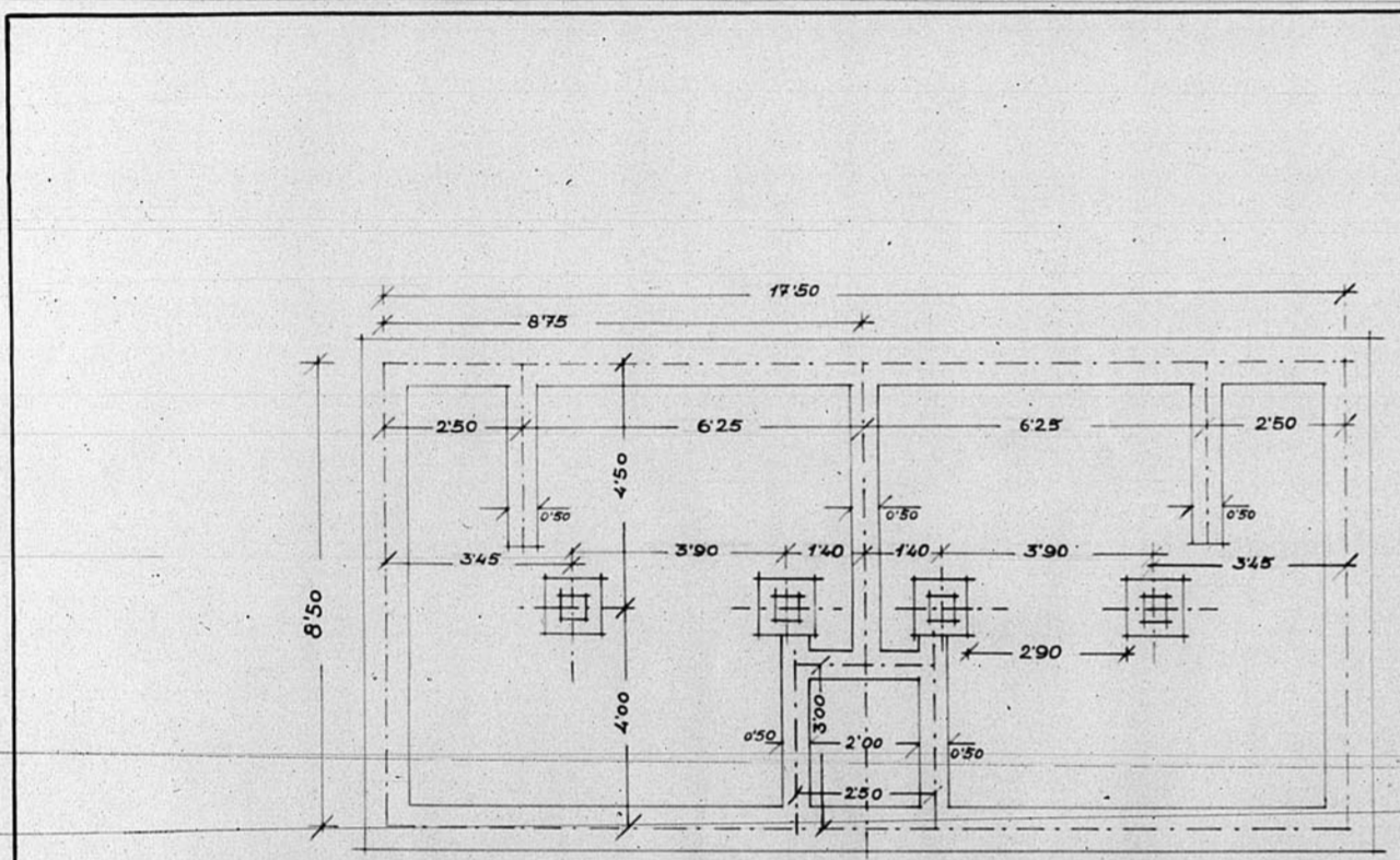
Cimientos
