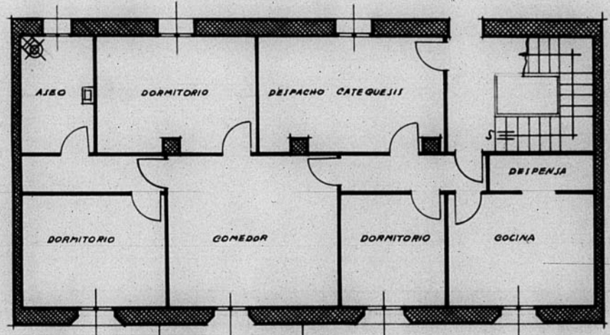
PLANTA 1ª
