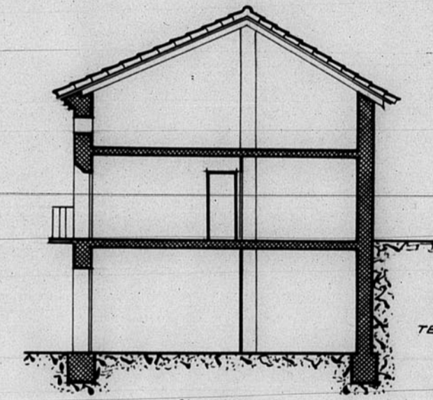
SECCION
