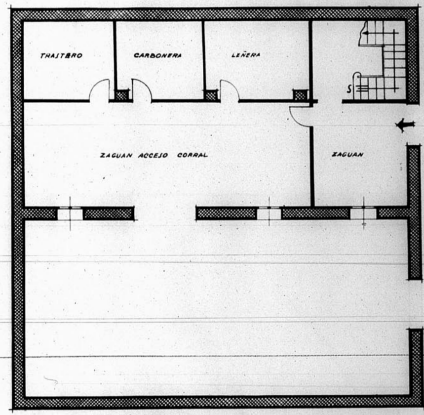
PLANTA BAJA
