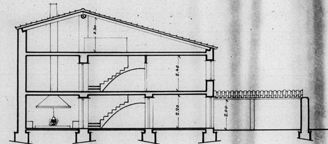
Sección A.B.
