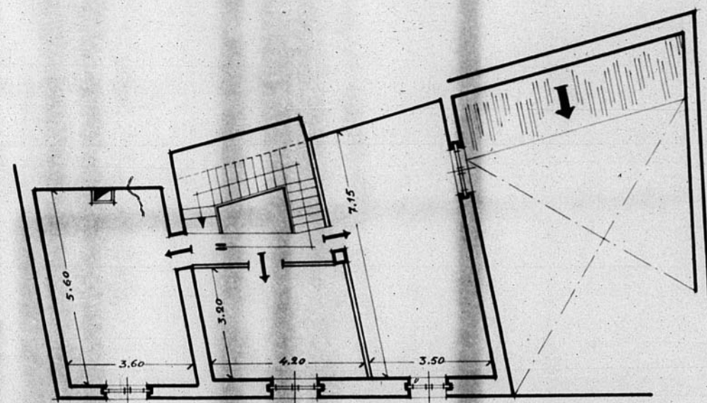
Planta primera
