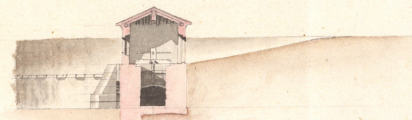
Figura 3.ª Perfil por las lineas EFGH.
