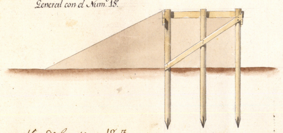
Figura 7.ª Perfil que manifiesta los Diques i ensamble de uno de los Diques de Madera y Corroyen q. se ha de construir en los parajes señalados en el Plano General con el Num. 18.
