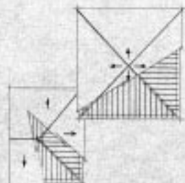
Planta de escaleras con dirección de movimiento y posición de la sección.
