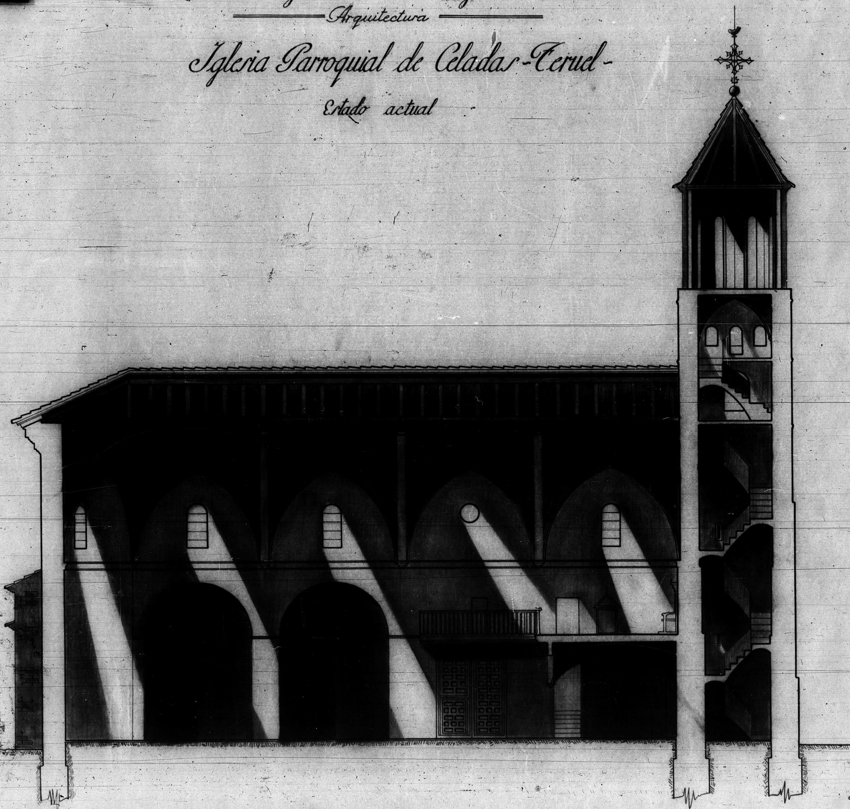
Sección Longitudinal
