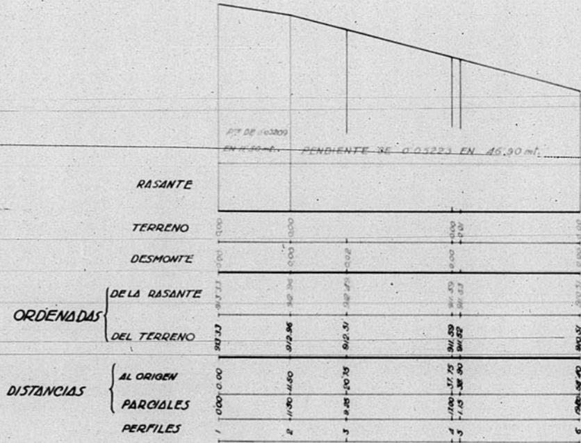
PERFIL LONGITUDINAL
