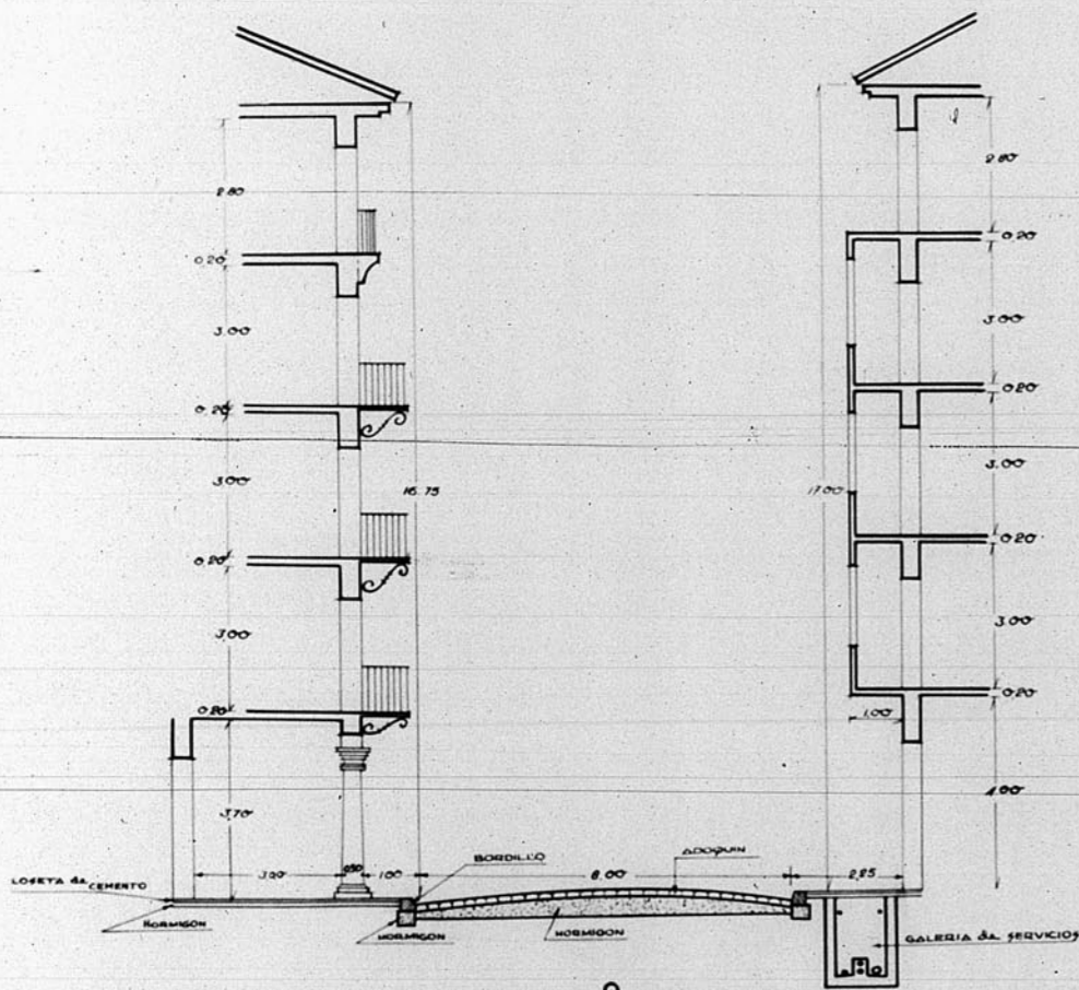
PERFIL TRANSVERSAL
