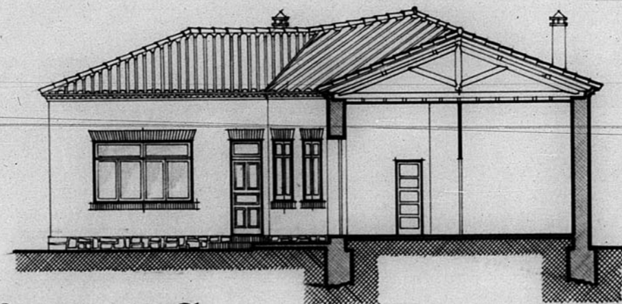
Sección A-B.
