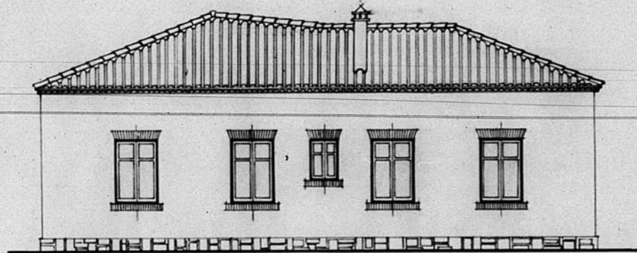
Alzado N.O.
