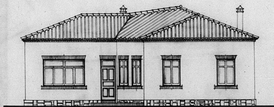
Alzado E.
