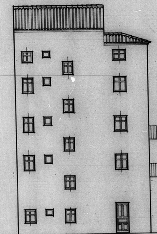
Fachada pral
