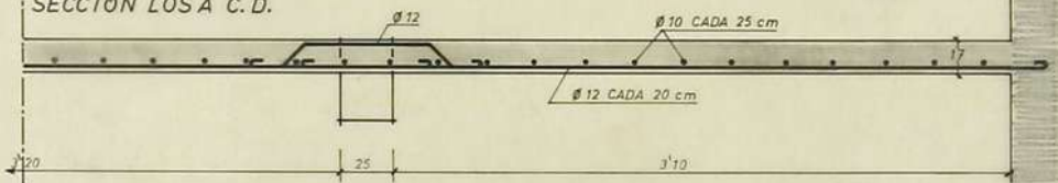
SECCIÓN LOSA C.D.
