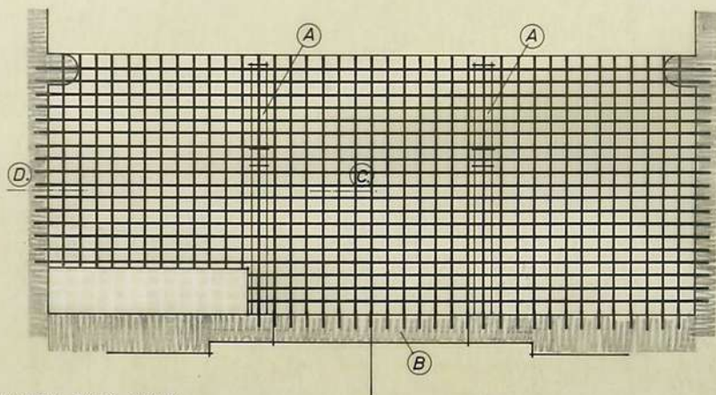
PLANTA PISO CORO
