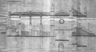
FACHADA LATERAL (CALLE DE PALACIO)
