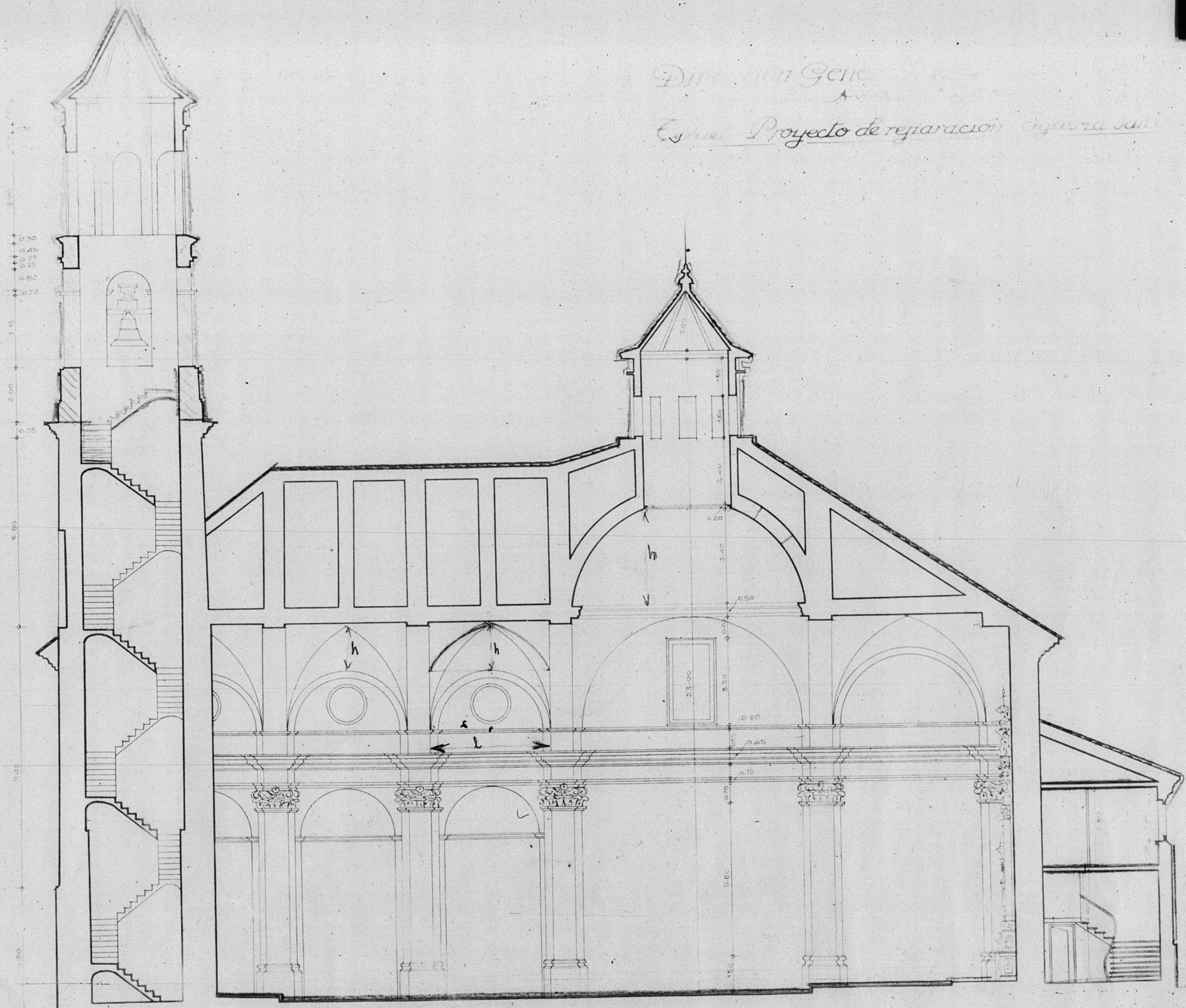
Sección longitudinal Escala 1:100
