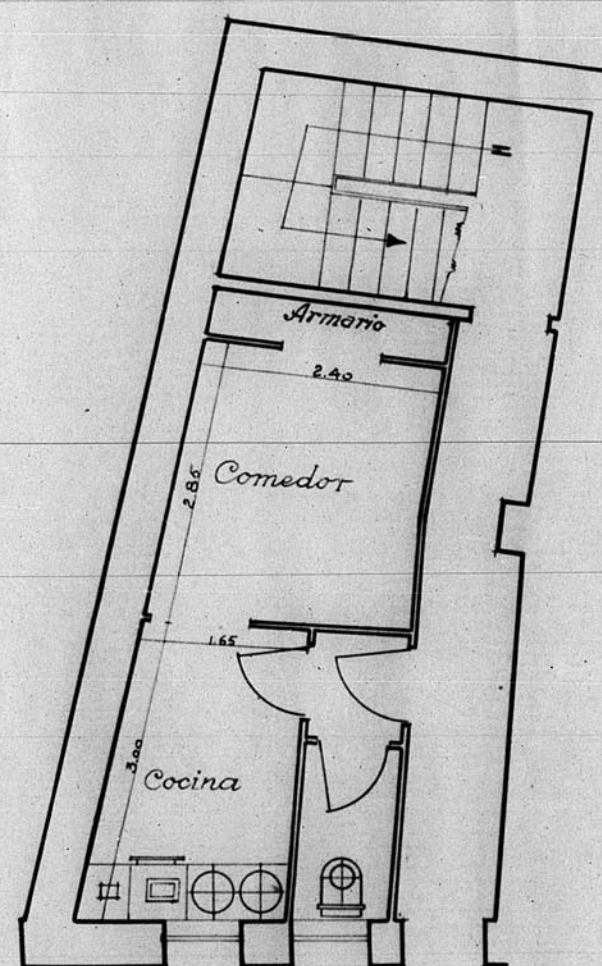
Planta baja
