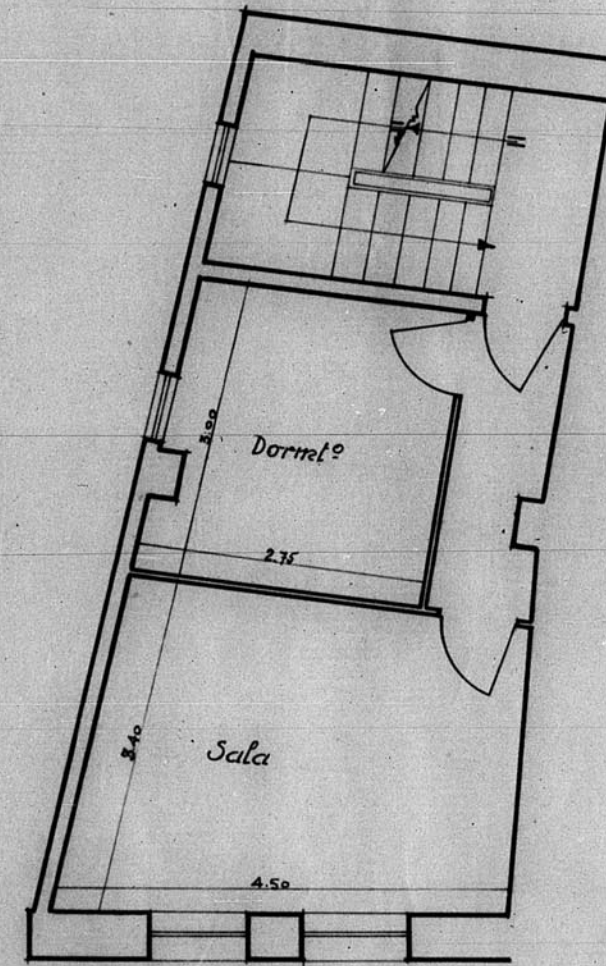
Planta 3ª
