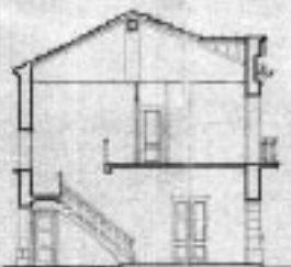
Sección
