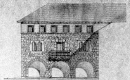
Alzado CD
