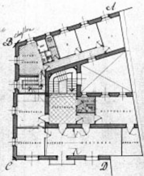
Planta 1ª
