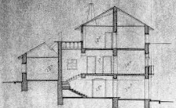
Sección EF
