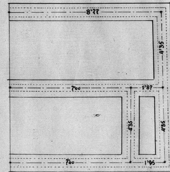
Cimientos
