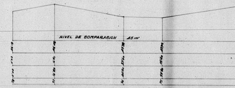
PERFIL J
