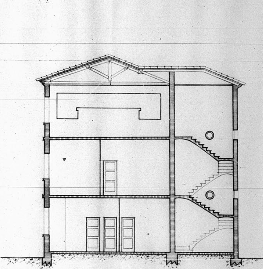
Sección A-B
