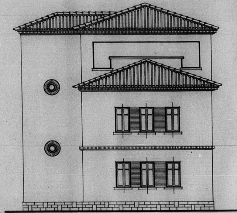
Alzado lateral
