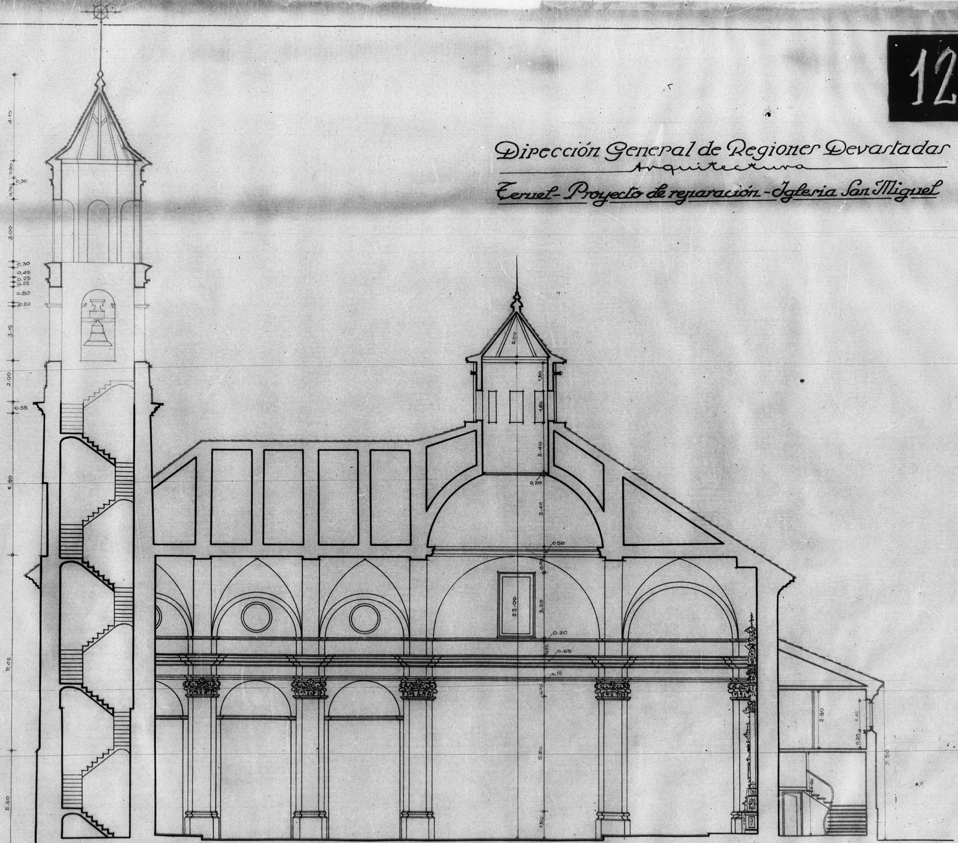
Sección Longitudinal Escala 1:100
