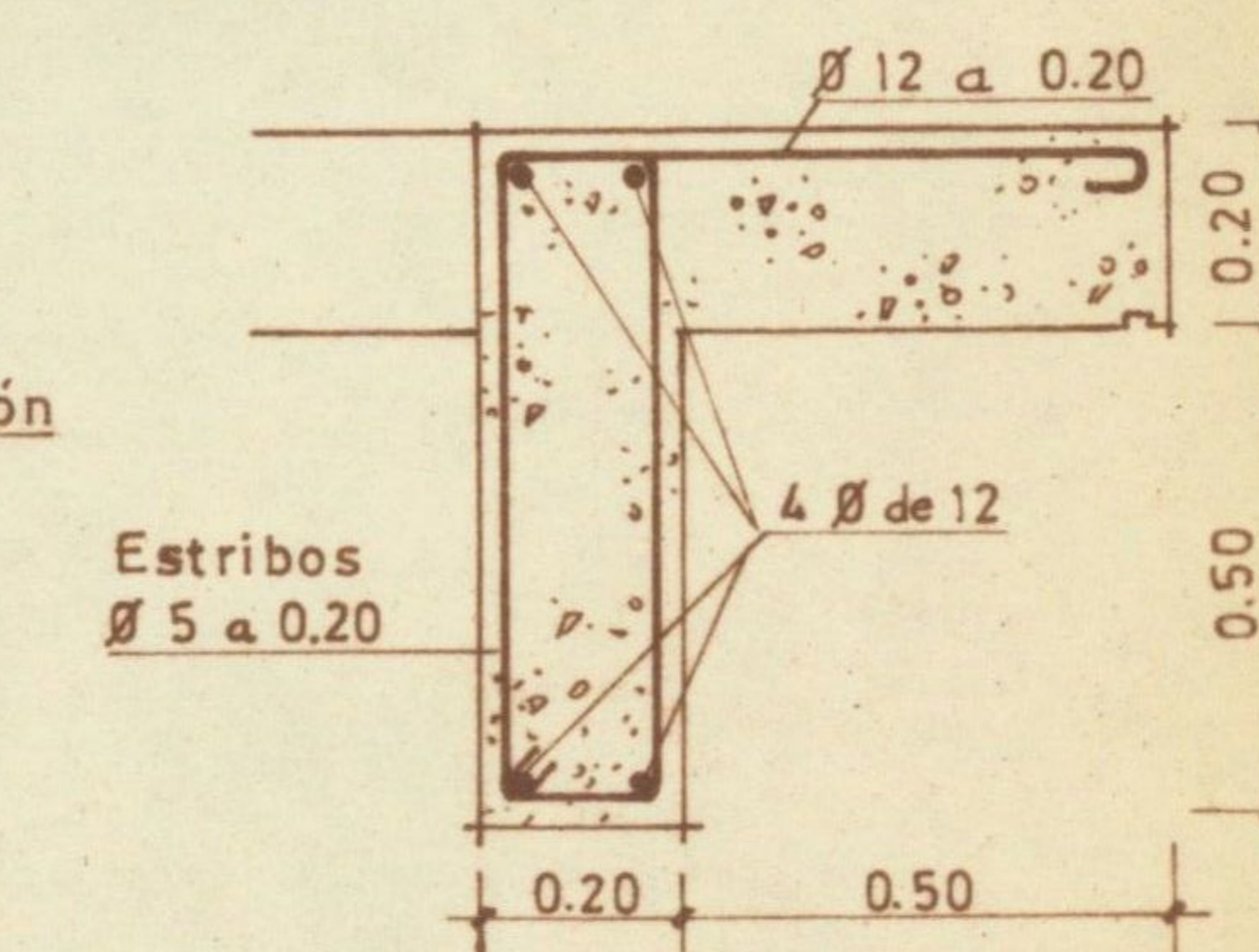
DETALLE B.
