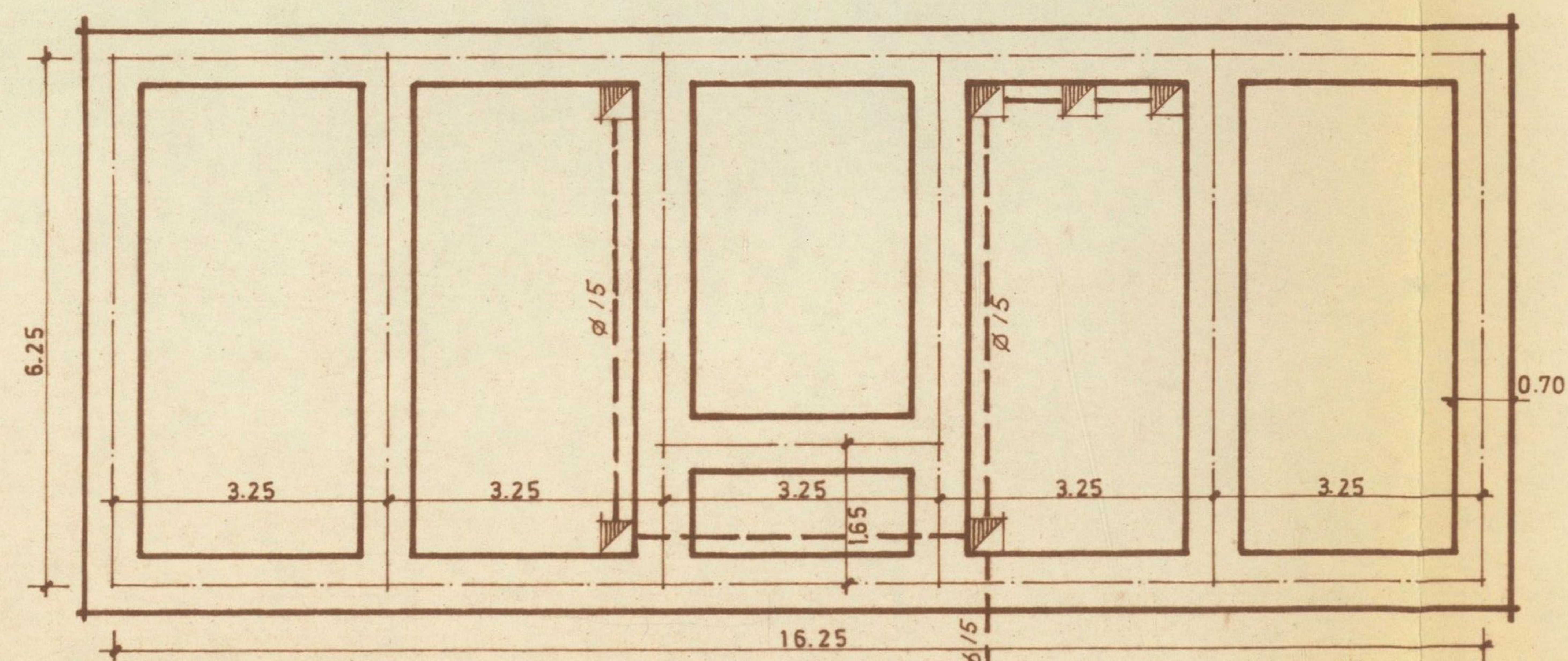
CIMIENTOS.
