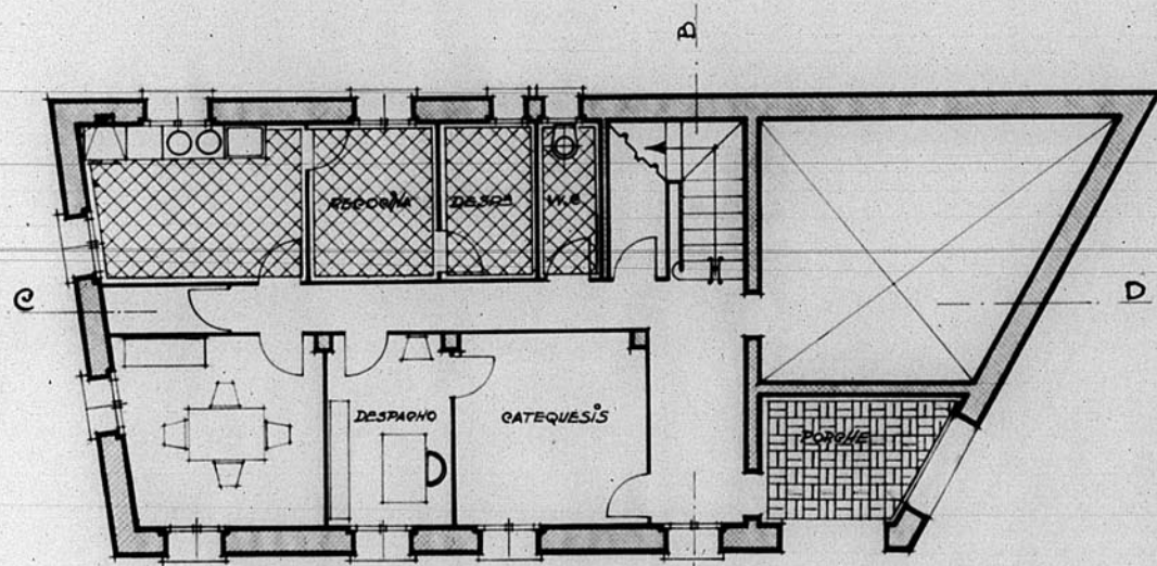
Planta baja.
