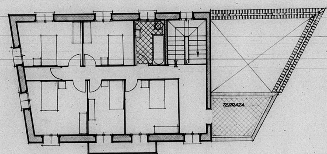
Planta 1ª.
