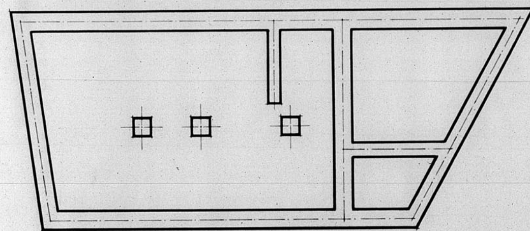
Cimientos.
