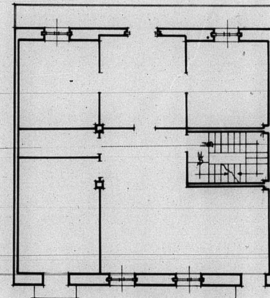
PLANTA 2ª
