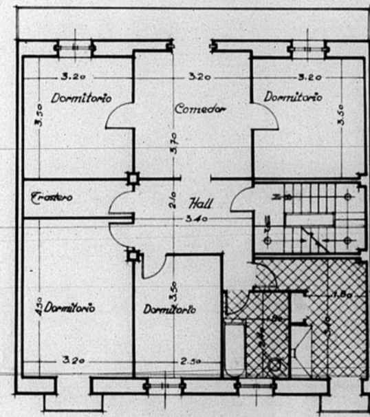
PLANTA 1ª
