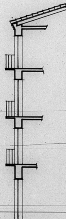
SECCION
