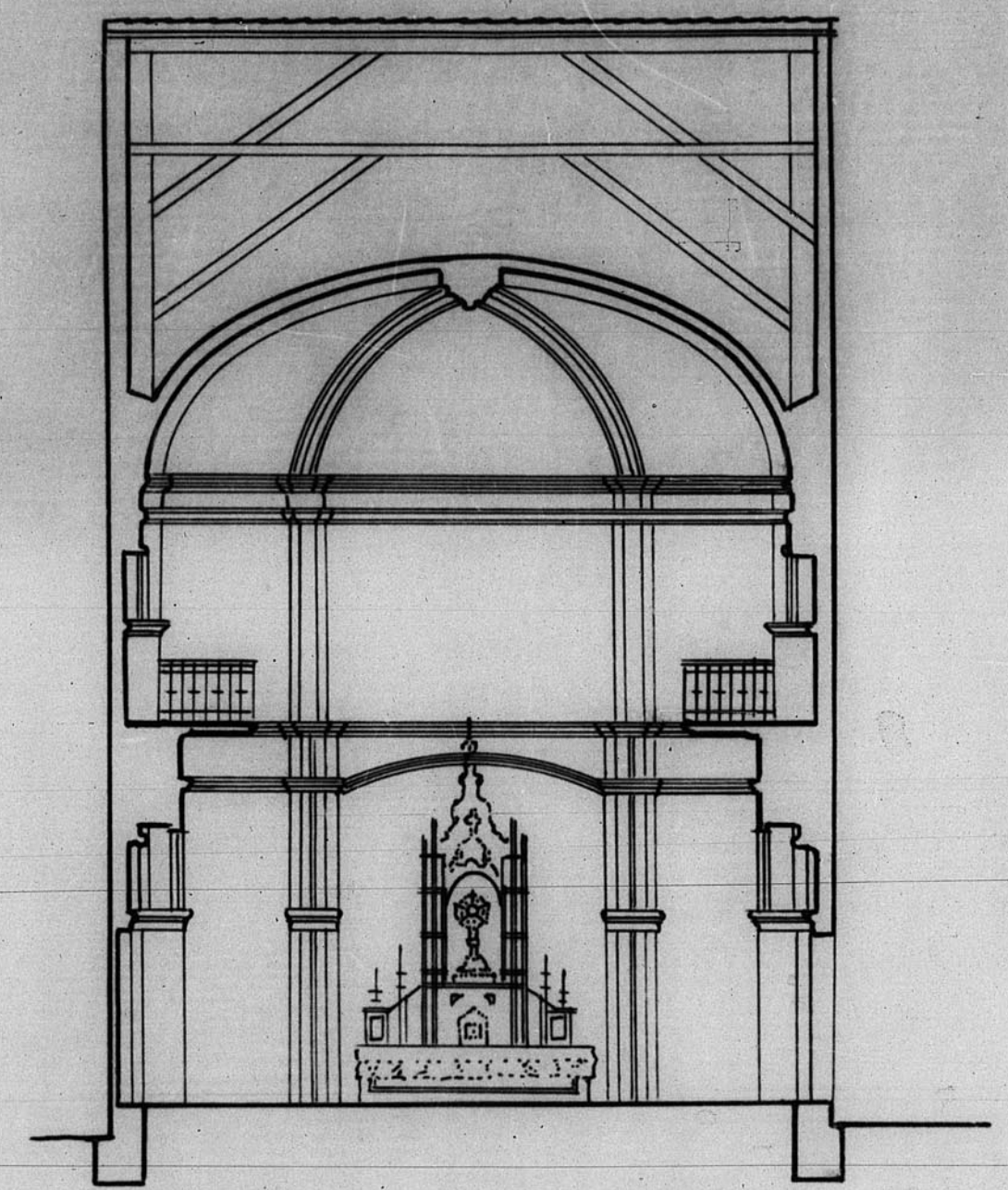
Sección C-D
