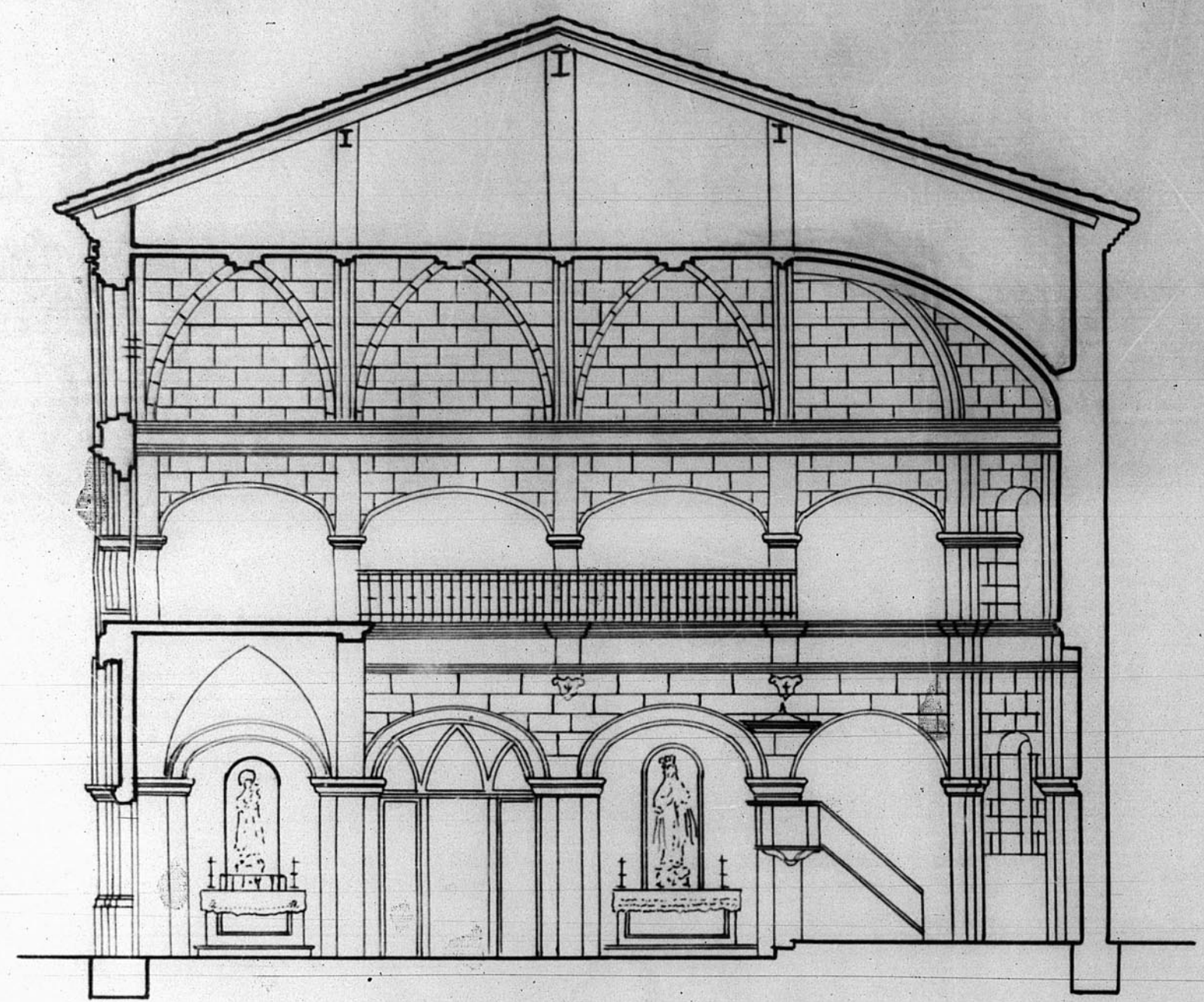
Sección A-B
