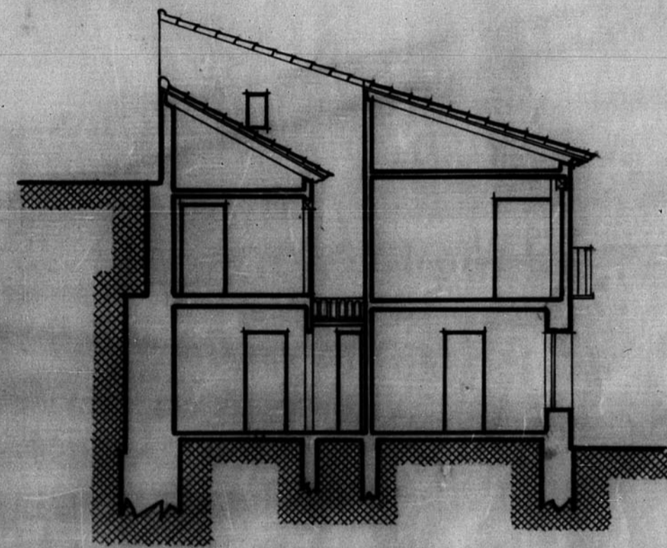
Sección A-B.
