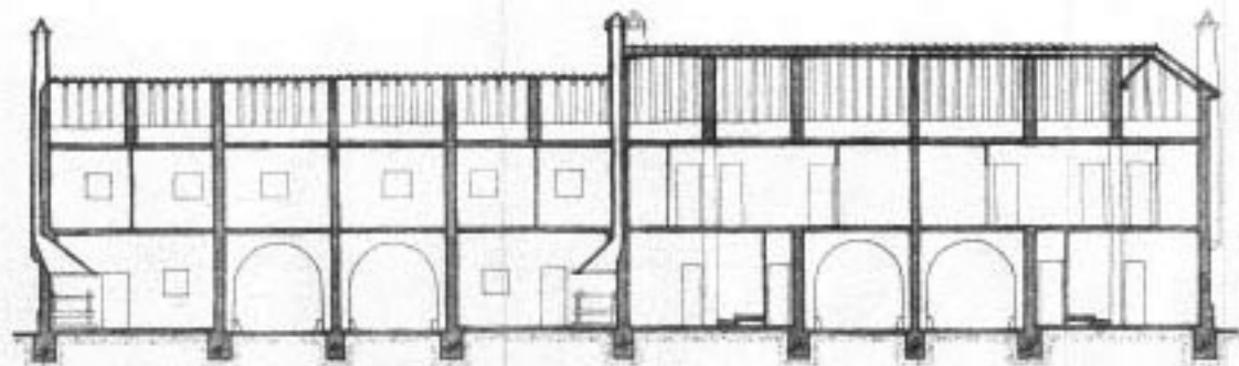
SECCIÓN A-B
