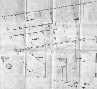
PLANTA BAJA ESCALA 1/50
