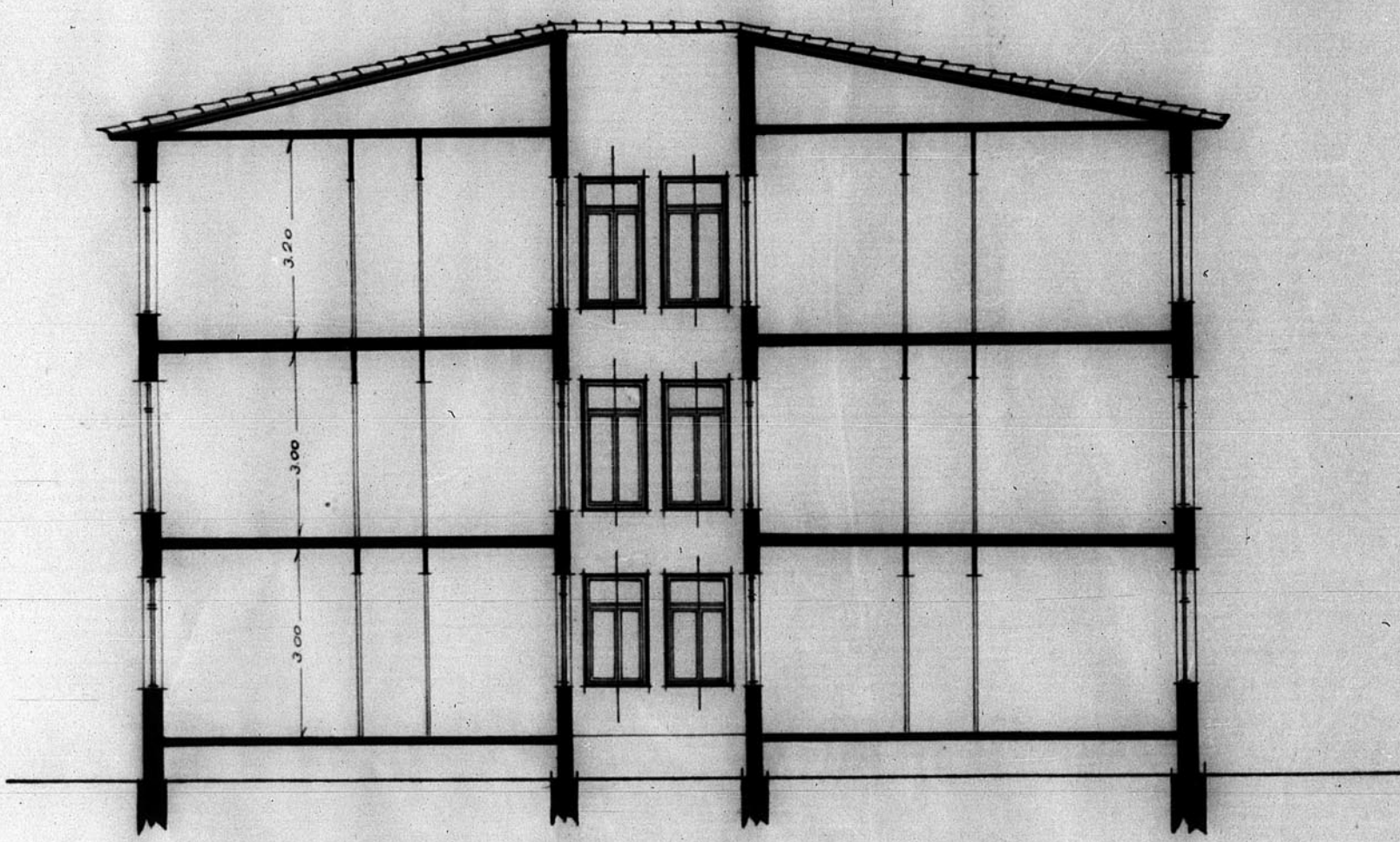
SECCION A-B
