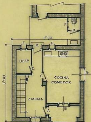
PLANTA BAJA
