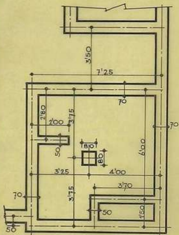
CIMENTOS
