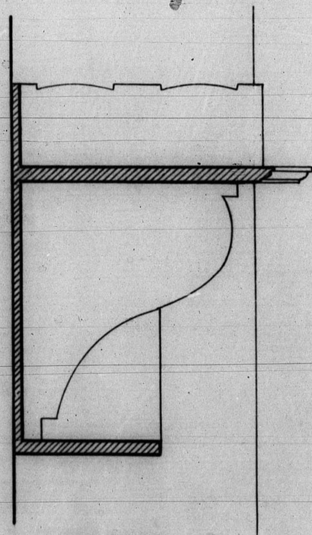
SECCION A.B.
