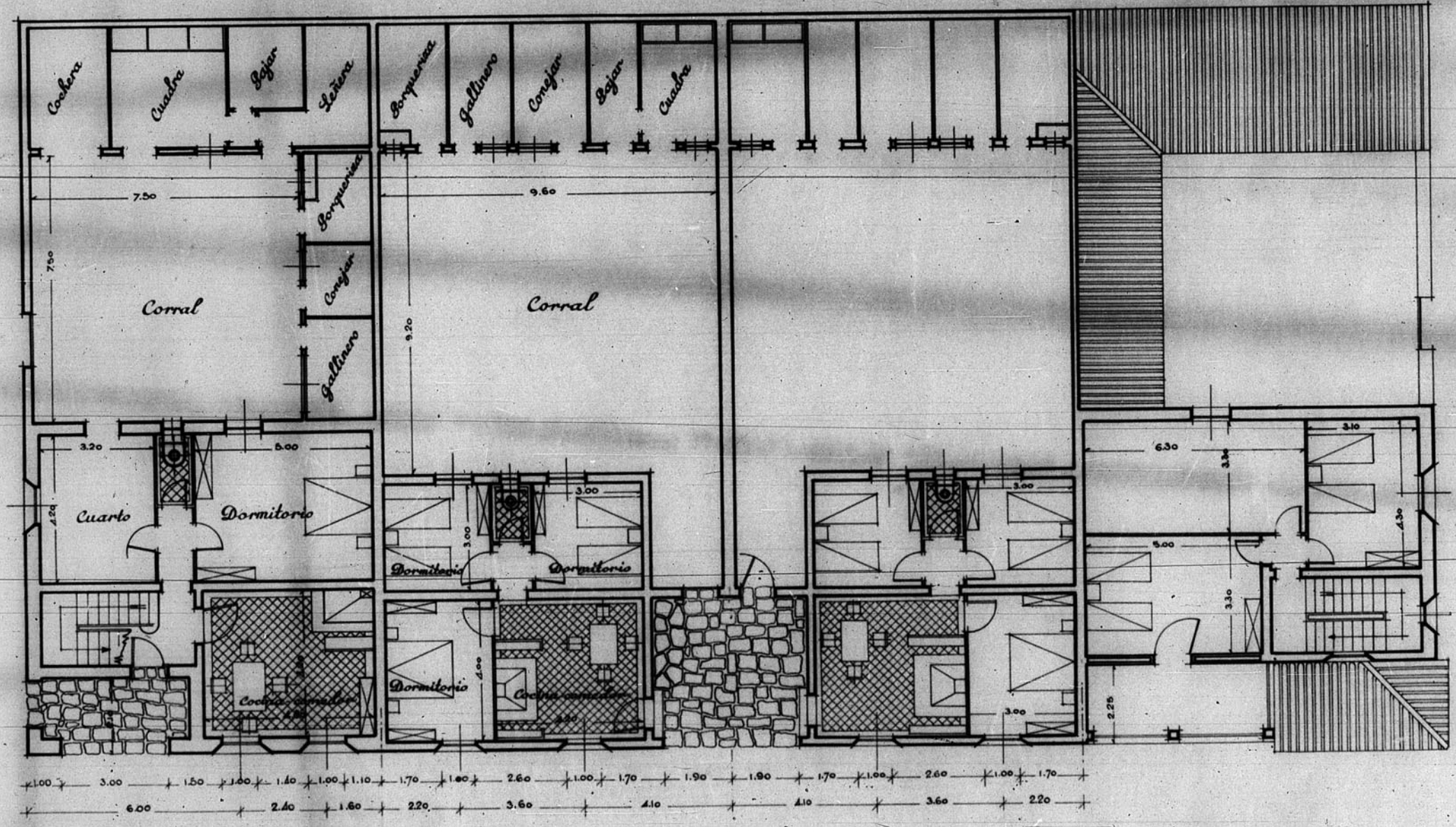
Planta baja
