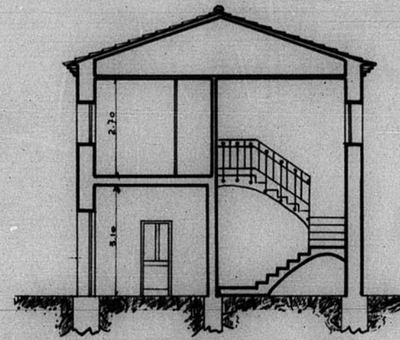
SECCION A-B
