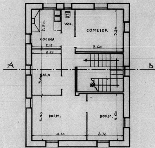
PLANTA 1ª
