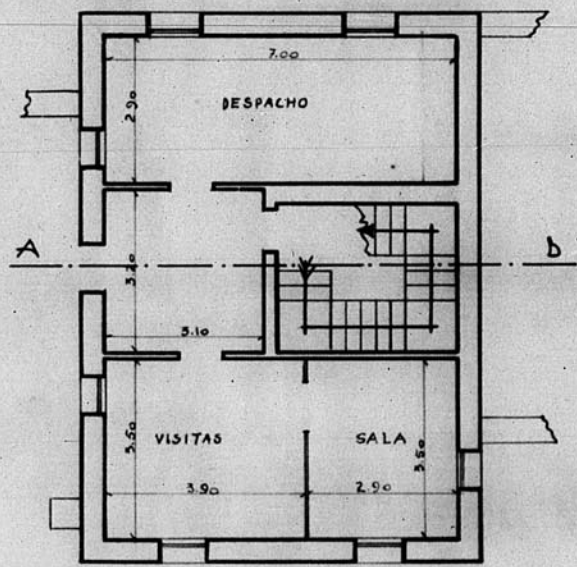
PLANTA DADA
