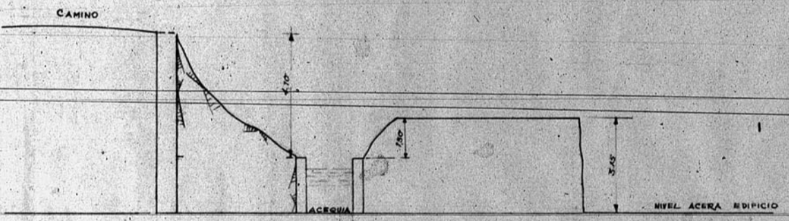
PERFIL A-B E = 1:100
