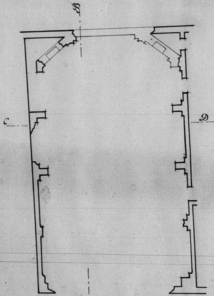
Planta baja
