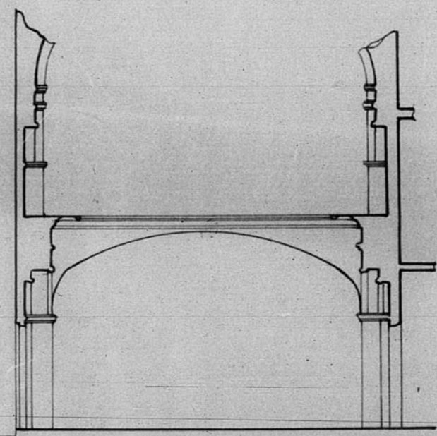
Sección C-D
