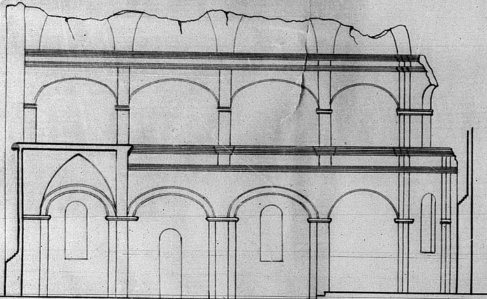
Sección A-B
