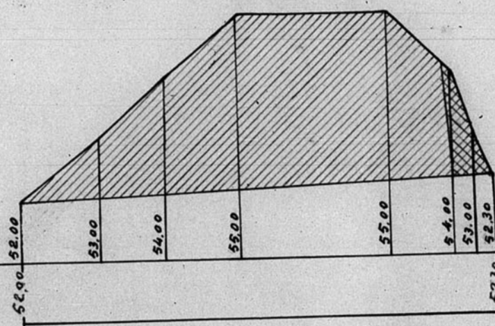
PERFIL nº 7-
