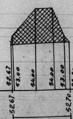
PERFIL nº 15-
