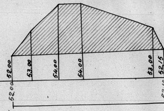
PERFIL nº 4-
