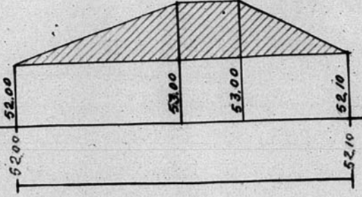
PERFIL nº 2-
