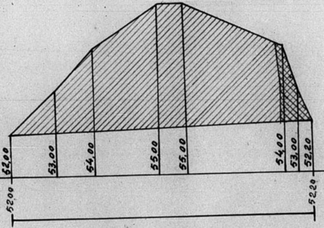
PERFIL nº 6-
