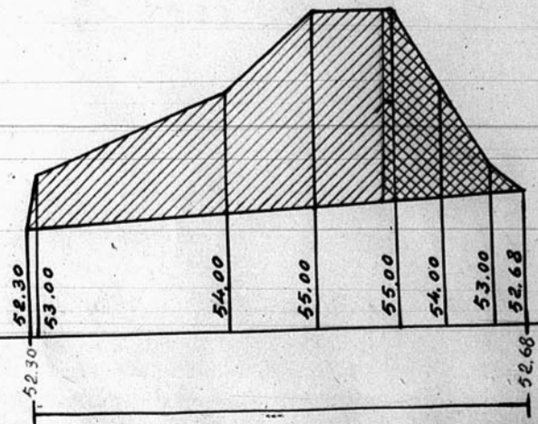
PERFIL nº 13-
