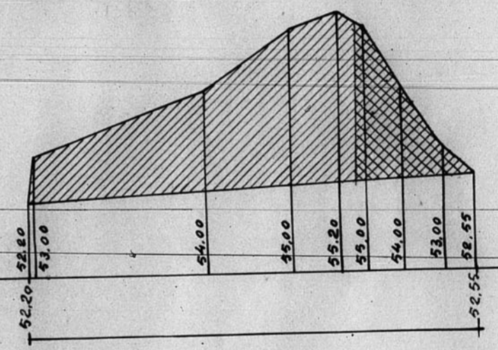
PERFIL nº 12-
