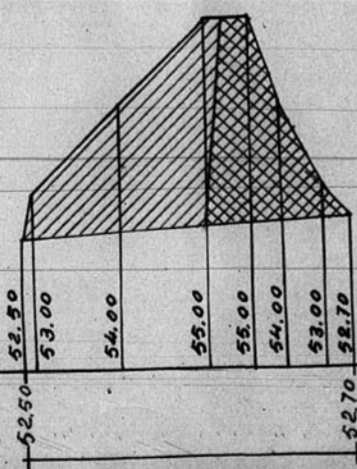
PERFIL nº 14-
