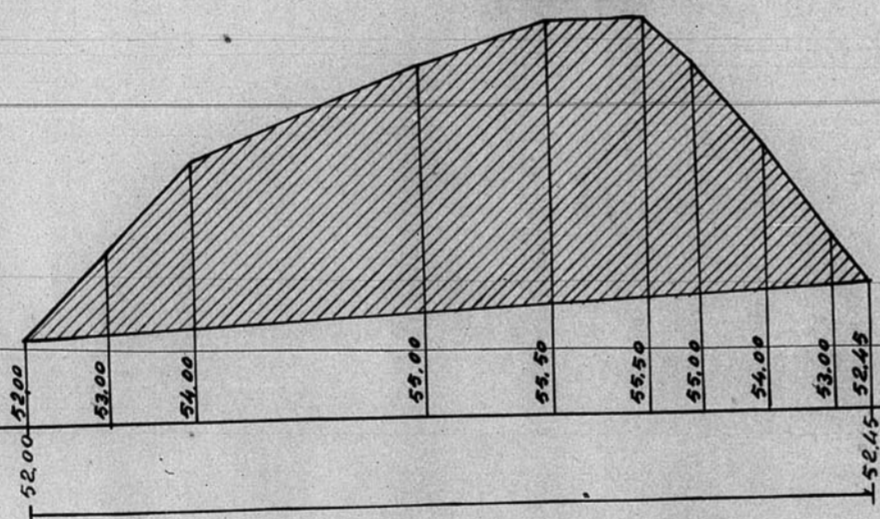
PERFIL nº 10-
