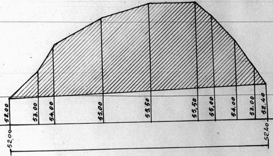
PERFIL nº 9-
