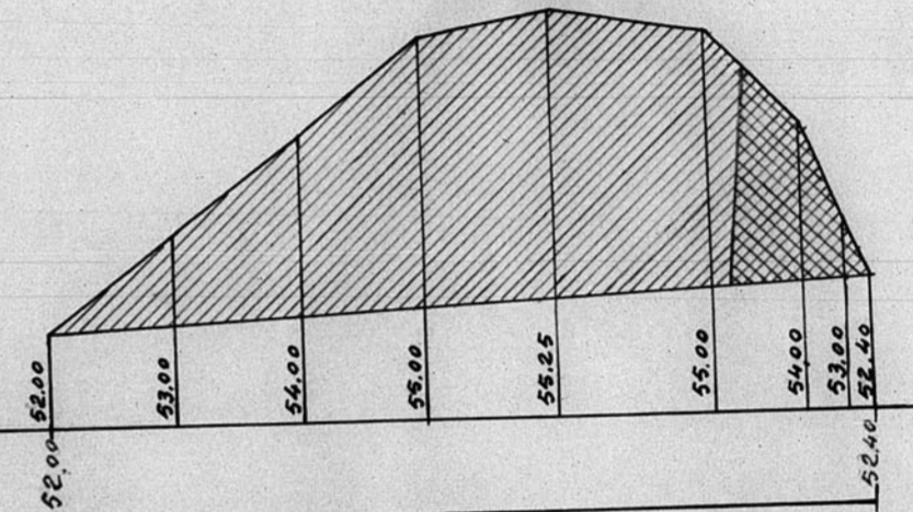
PERFIL nº 8-
