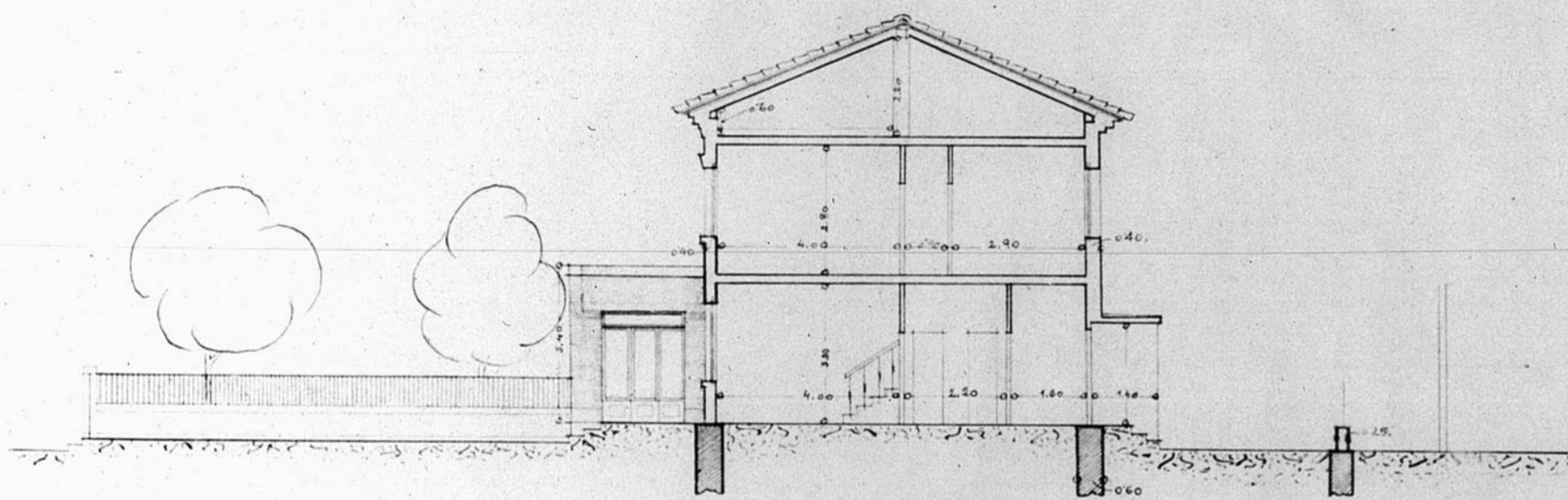
Sección A-D.
