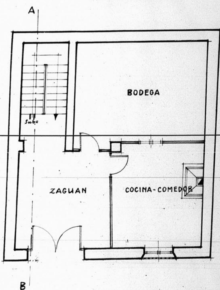
PLANTA BAJA
