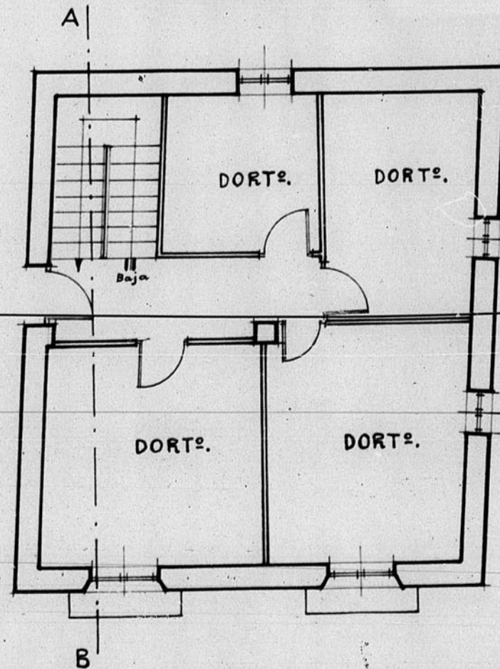
PLANTA 1ª
