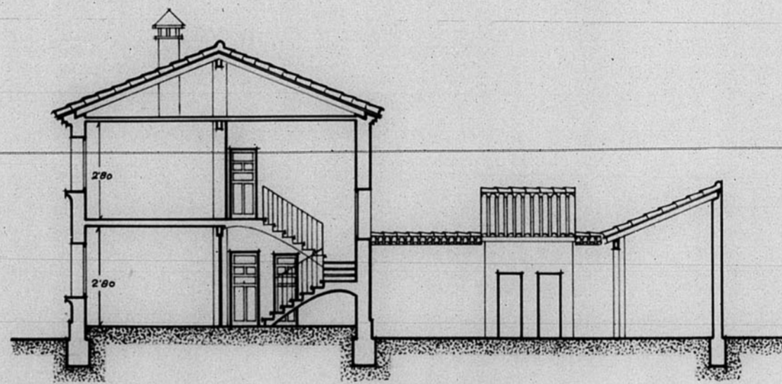
Sección
