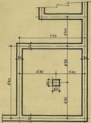
CIMENTOS
