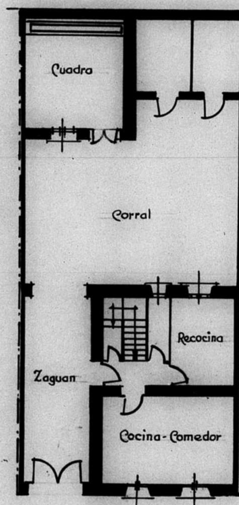
PLANTA BAJA
