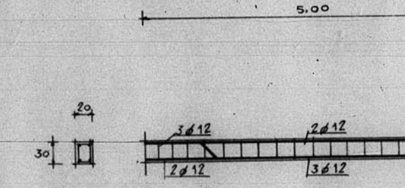
VIGA 6-13 TIPO ② 20x30
