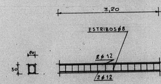
VIGAS 18-19, 16-11, 15-10 y 7-8 TIPO ① 20x30
