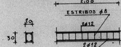
VIGAS 18-17 y 19-12 TIPO ① 20x30
