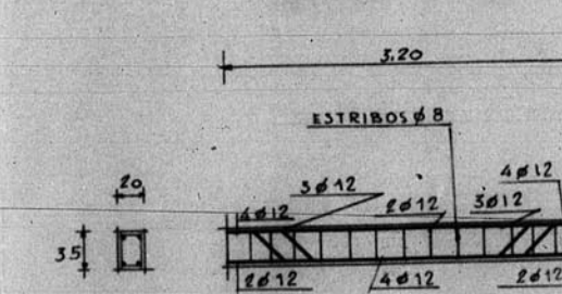
VIGA 14-9 TIPO ⑤ 20x35
