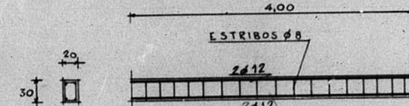
VIGAS 16-15 y 11-10 TIPO ① 20x30
