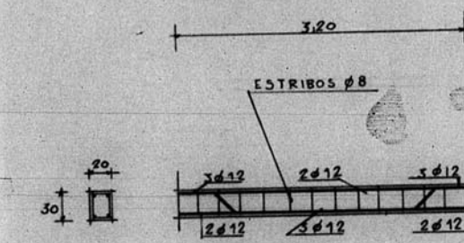
VIGA 17-12 TIPO ② 20x30
