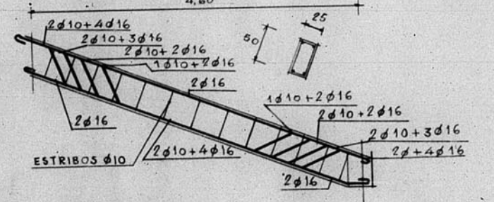
VIGA F-6 TIPO ② 25x50
