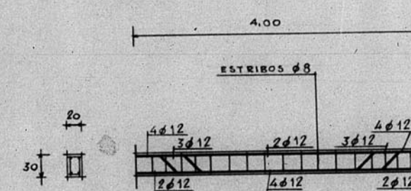
VIGAS 17-16, 12-11, 15-14 y 10-9 TIPO ③ 20x30
