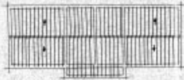
Faja de cubierta Columbros y vigas de hormigón pretensado.
