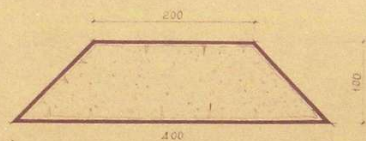
DIQUE DE TIERRA (SECCION PROYECTADA)
