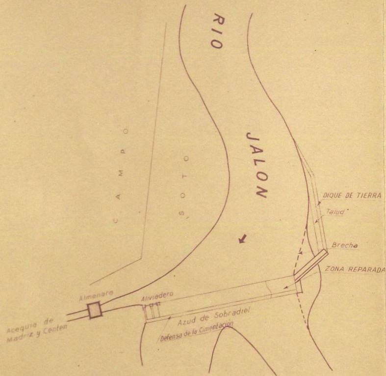
PLANTA ESCALA 1:1000
