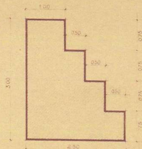
DIQUE DE TIERRA (SECCION PROYECTADA)
