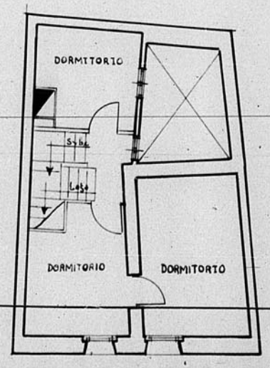
Planta 1ª
