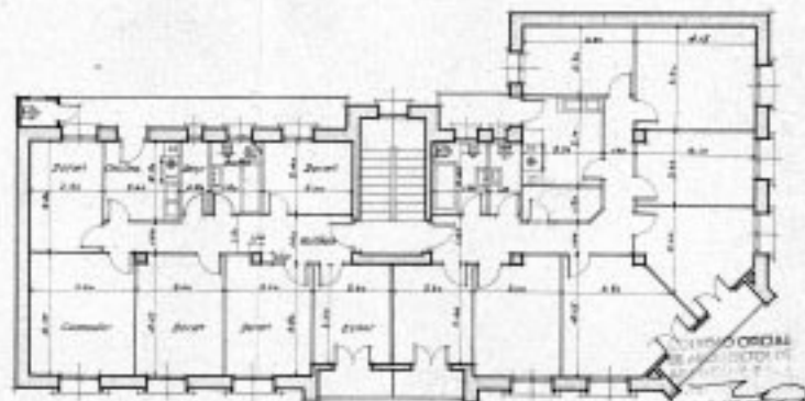
Planta de pisos
