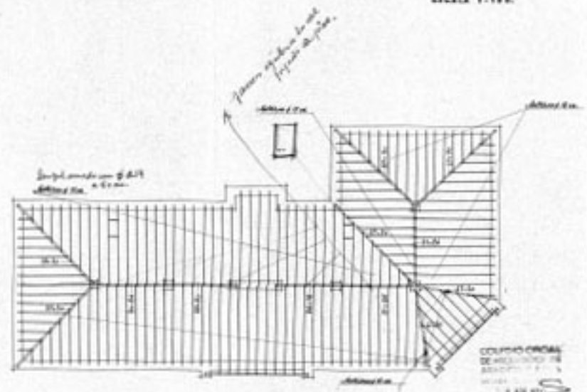
Planta de Estructura de Cubiertas
