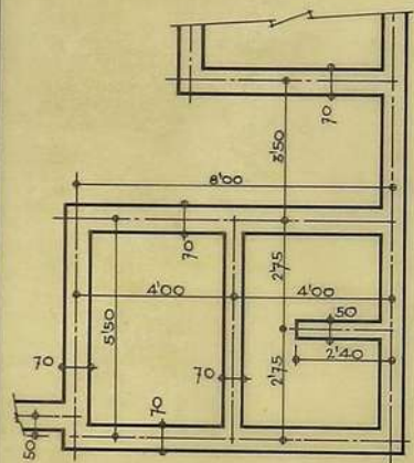
CIMENTOS
