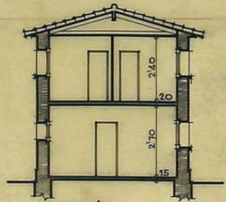
SECCIÓN
