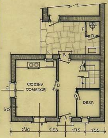
PLANTA BAJA
