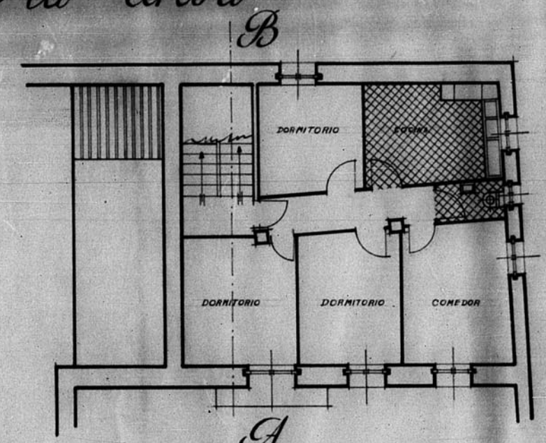
Planta 1ª
