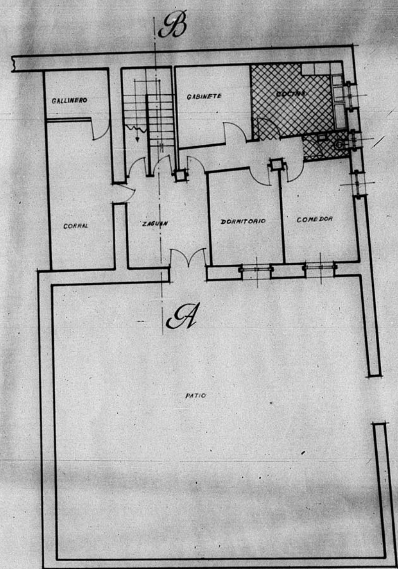
Planta baja
