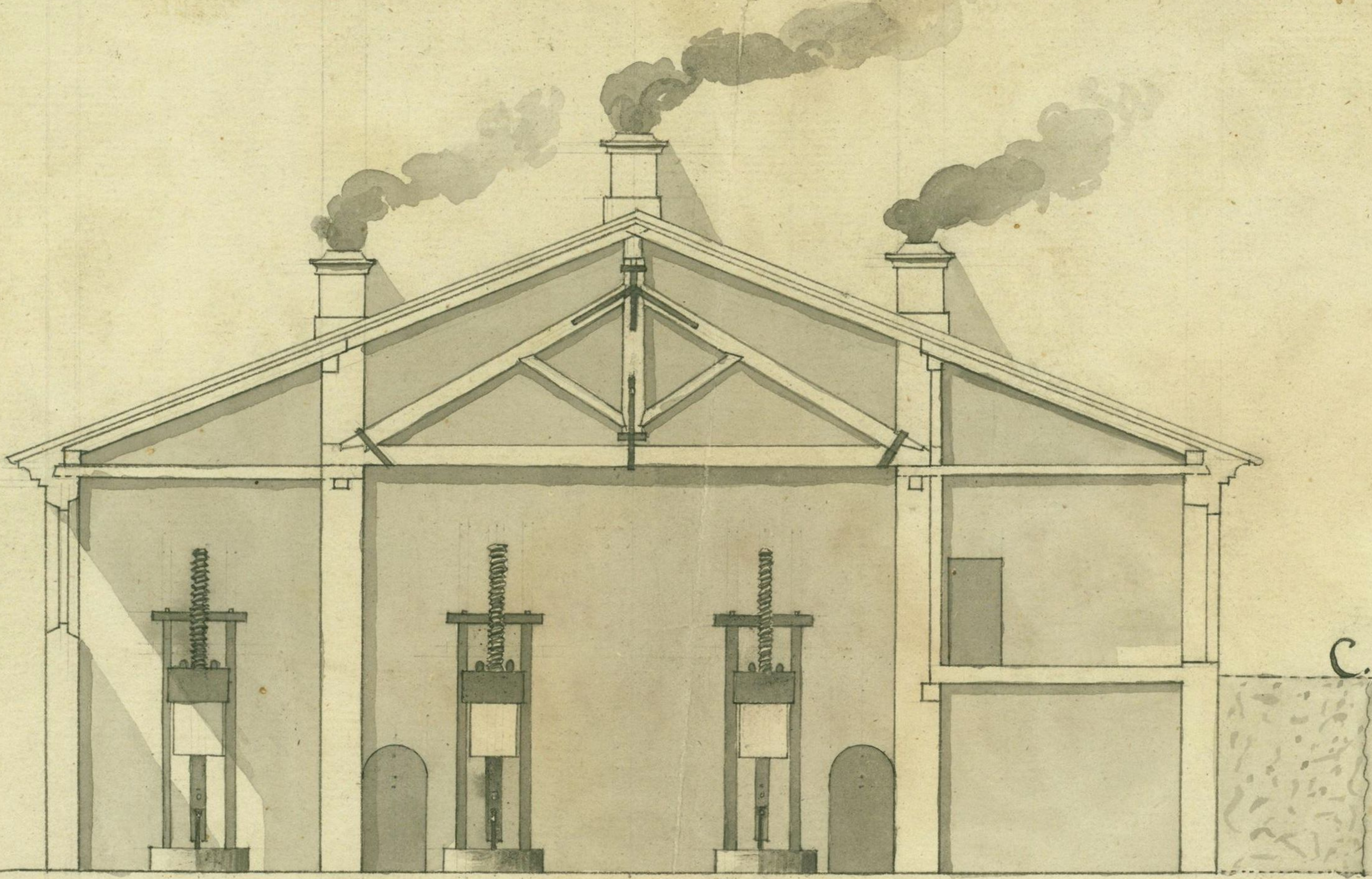
Perfil Levantado Sobre la Línea. AB de la Planta.
